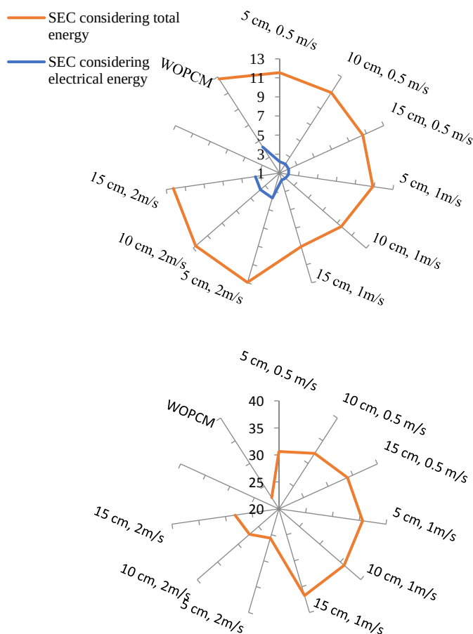
شکل ۱۰- الف). مقادیر SEC (با در نظر گرفتن انرژی الکتریکی و انرژی کل)، ب) راندمان کلی خشک کردن خورشیدی سنج در شرایط مختلف جریان هوا و فواصل مواد تغییر فازدهنده
