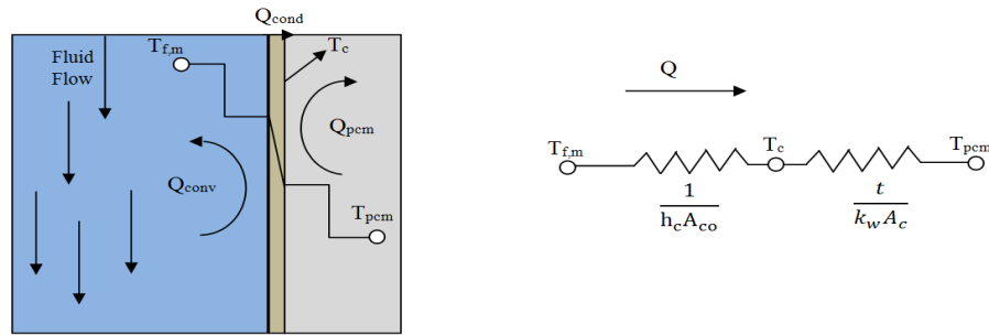
شکل ۳- مدار انتقال حرارت برای سیال، لوله مسی و پارافین به عنوان ماده PCM Fig. 3. Heat transfer circuit for fluid, copper tube and paraffin as PCM material
