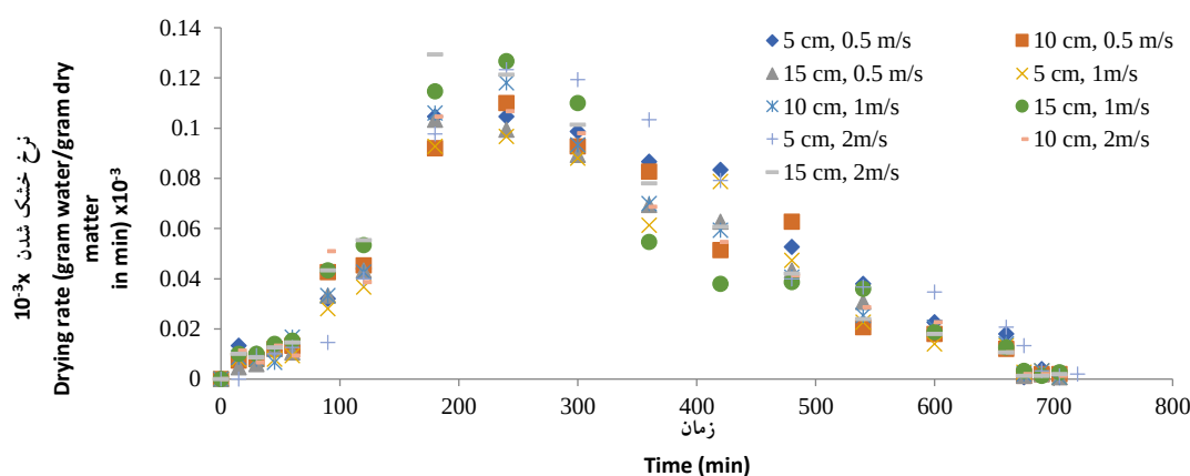
شکل ۹- تغییرات نرخ خشک شدن میوه سنجید با زمان در فواصل مختلف لوله‌ها با سرعت‌های مختلف
