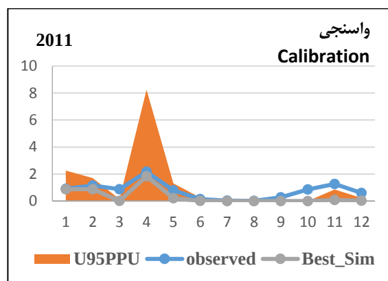
شکل ۹- منحنی رابطه رواناب مشاهده‌ای و شبیه‌سازی شده منطقه در دوره واسنجی ۲۰۰۲-۲۰۰۹
