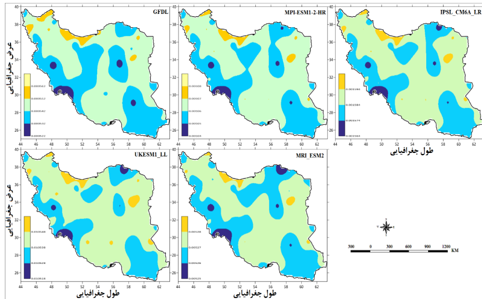
شکل ۳- خطای RMSE بارش برآورد شده از طریق مدل‌های مختلف Fig.3. RMSE error of estimated precipitation from different models
