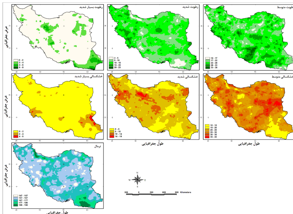
شکل ۱۰- فراوانی رخداد انواع وضعیت SPEI طی دوره ۲۰۴۰ – ۲۰۲۱ بر اساس سناریوی SSP5-8.5
