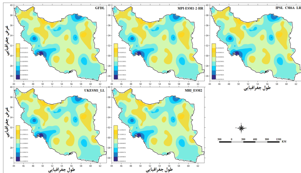
شکل ۴- خطای MAE بارش برآورد شده از طریق مدل‌های مختلف Fig.4. MAE error of estimated precipitation from different models
