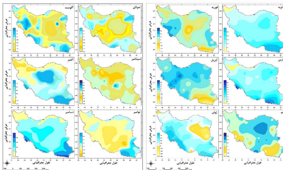
شکل ۹- درصد ناهنجاری بارش ماه‌های ژانویه تا دسامبر دوره آینده نزدیک بر اساس سناریوی SSP5-8.5 Fig.9. Percentage anomaly of precipitation from January to December in the near future period based on the SSP5-8.5 scenario
