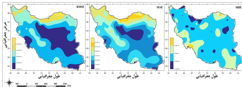
شکل ۶- خطاهای مختلف بارش همادی شده ی مدل‌های مختلف
