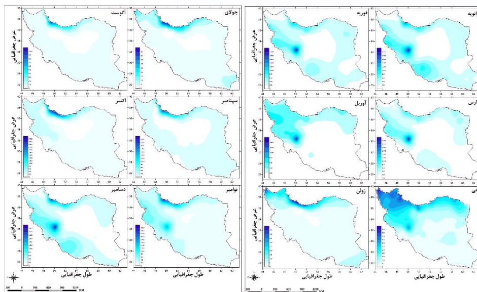
شکل ۷- نقشه میانگین مجموع بارش ماه‌های ژانویه تا دسامبر دوره آماری ۱۹۸۵ - ۲۰۱۴
