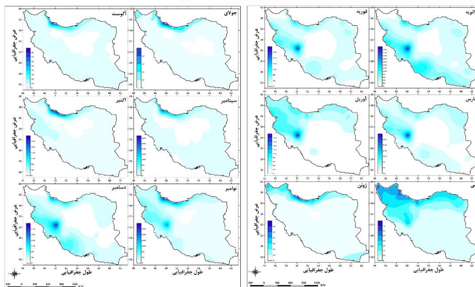
شکل ۸- نقشه میانگین مجموع بارش ماه های ژانویه تا دسامبر دوره آماری ۲۰۴۰ - ۲۰۲۱ بر اساس سناریوی SSP5-8.5 Fig.8. Map of average total precipitation from January to December during the statistical period 2021–2040 based on the SSP5-8.5 scenario
