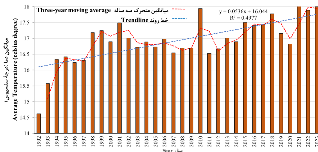
شکل ۳- میانگین سالانه دما در ایران
