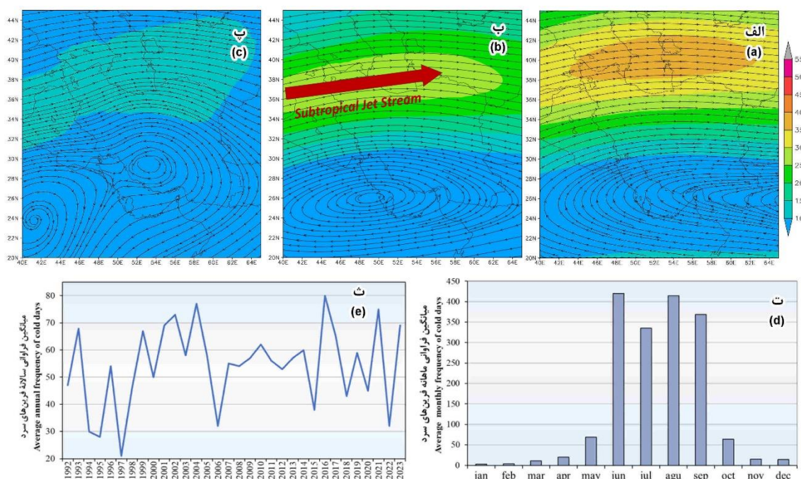
شکل ۱۰- خوشه شش: الف) جریان باد تراز ۲۰۰ هکتوپاسکال ( \text{m}\cdot\text{s}^{-1} )، ب) جریان باد تراز ۳۰۰ هکتوپاسکال ( \text{m}\cdot\text{s}^{-1} )، پ) جریان باد تراز ۵۰۰ هکتوپاسکال ( \text{m}\cdot\text{s}^{-1} )، ت) میانگین فراوانی ماهانه و ث) میانگین فراوانی سالانه فرین‌های سرد در بازه ۳۲ ساله در ایران
