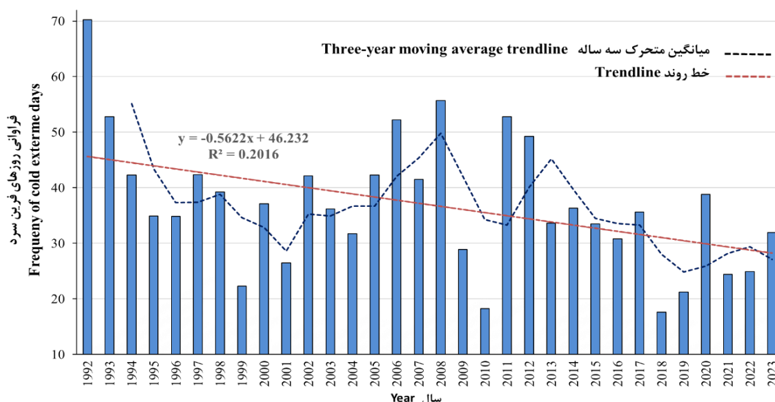
شکل ۲- میانگین فراوانی سالانه رویدادهای فرین سرد در ایران
