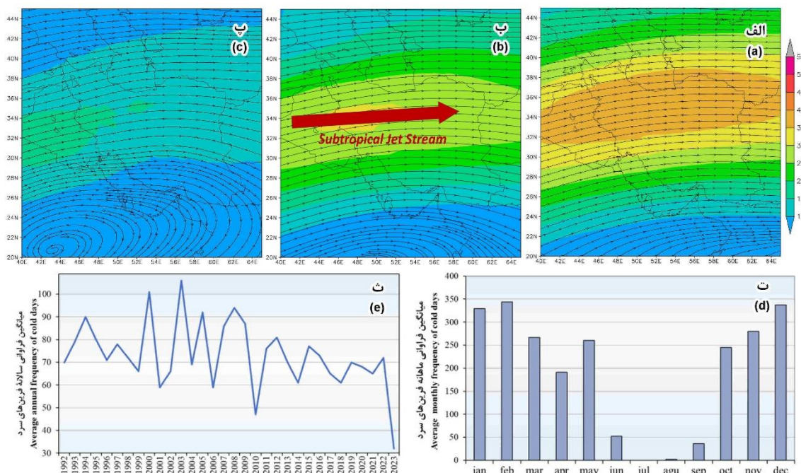
شکل ۸- خوشه پنج: الف) جریان باد تراز ۲۰۰ هکتوپاسکال ( m \cdot s^{-1} )، ب) جریان باد تراز ۳۰۰ هکتوپاسکال ( m \cdot s^{-1} )، پ) جریان باد
