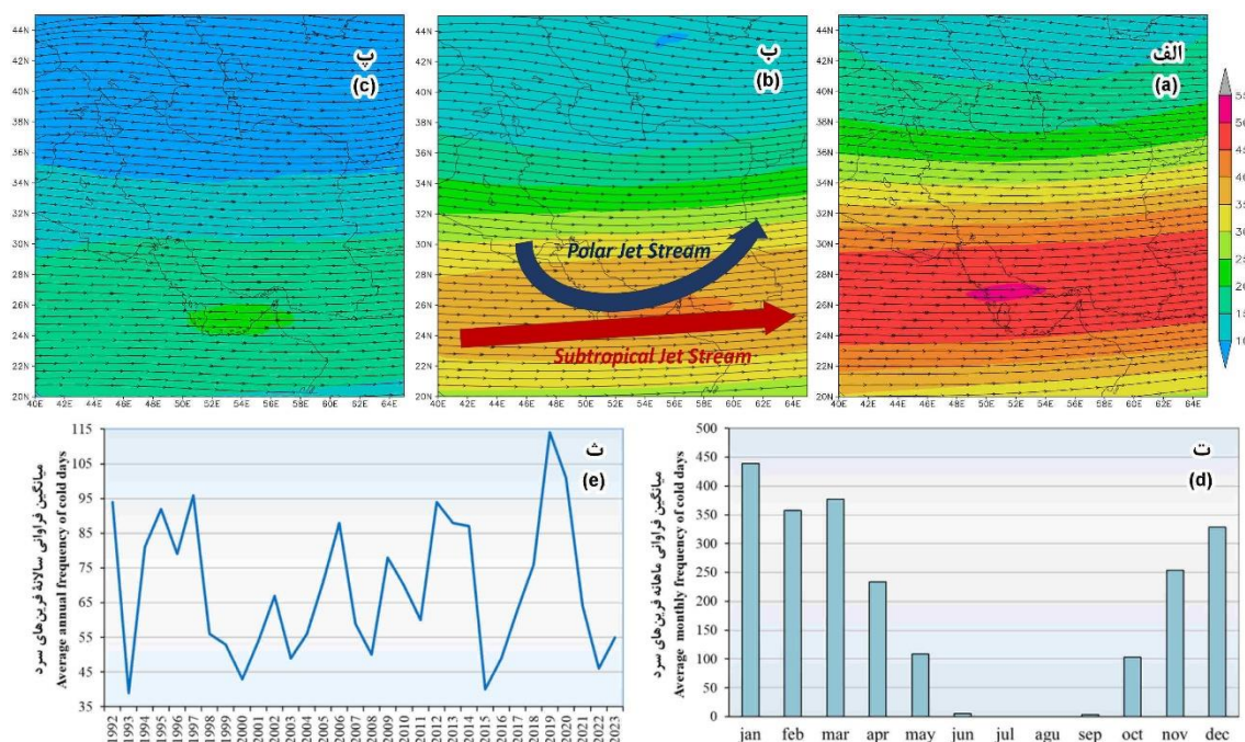
شکل ۵- خوشه یک: الف) جریان باد تراز ۲۰۰ هکتوپاسکال ( m \cdot s^{-1} ), ب) جریان باد تراز ۳۰۰ هکتوپاسکال ( m \cdot s^{-1} ), پ) جریان باد تراز
