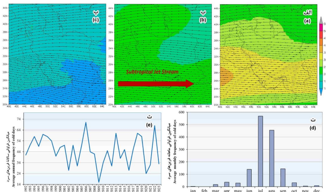
شکل ۷- خوشه دو: الف) جریان باد تراز ۲۰۰ هکتوپاسکال ( m \cdot s^{-1} )، ب) جریان باد تراز ۳۰۰ هکتوپاسکال ( m \cdot s^{-1} )، پ) جریان باد
