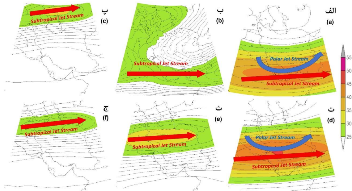
شکل ۴- خوشه‌های باد تراز ۳۰۰ هکتوپاسکال (ارقام بر حسب متربرثانیه؛ الف خوشه یک، ب خوشه دو، پ خوشه سه، ت خوشه چهار، ث خوشه پنج، ج خوشه شش
