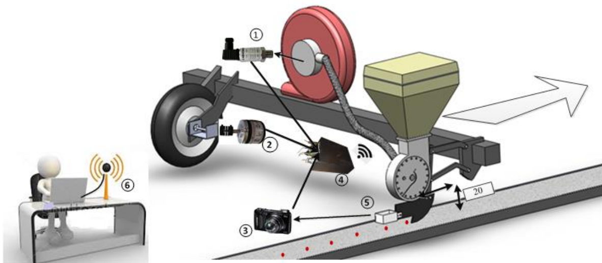
شکل ۱- شماتیک تجهیز بذرکار به ابزار دقیق: (۱) ترانسمیتر، (۲) دورسنج نوری، (۳) دوربین سرعت بالا، (۴) واحد پردازش مرکزی، (۵) محل قرارگیری دوربین، (۶) سیستم نظارت
