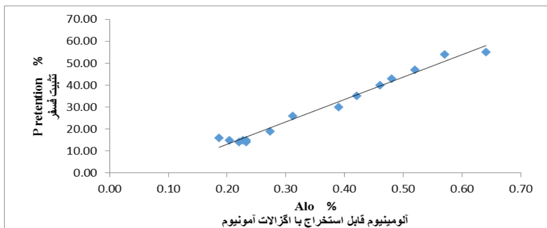
شکل ۴- همبستگی ( r : +/0.99^{**} ) بین درصد تثبیت فسفر با درصد آلومینیوم قابل استخراج با اگزالات آمونیوم در خاک‌های مورد مطالعه (۱ و ۳۲) Figure 4- Correlation ( r : 0.99^{**} ) between P retention percentage and ammonium oxalate extractable Al in the studied soils
