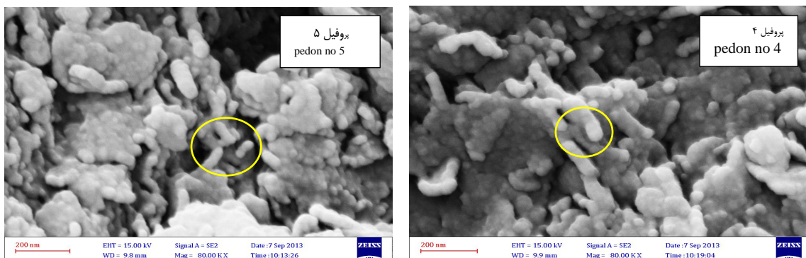
شکل ۳- نانوگراف تهیه شده از نانوذرات آلوپانی پروفیل چهار (راست) و پروفیل پنج (چپ) توسط میکروسکوپ الکترونی روبشی (۳۲) Figure 3- Nanographs prepared from Allophanic nanoparticles pedon no 4 (right) and pedon no 5 (left) by SEM
